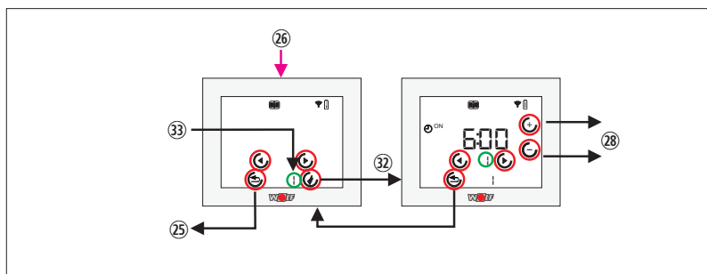
Рис. 10.16 Недельная программа
