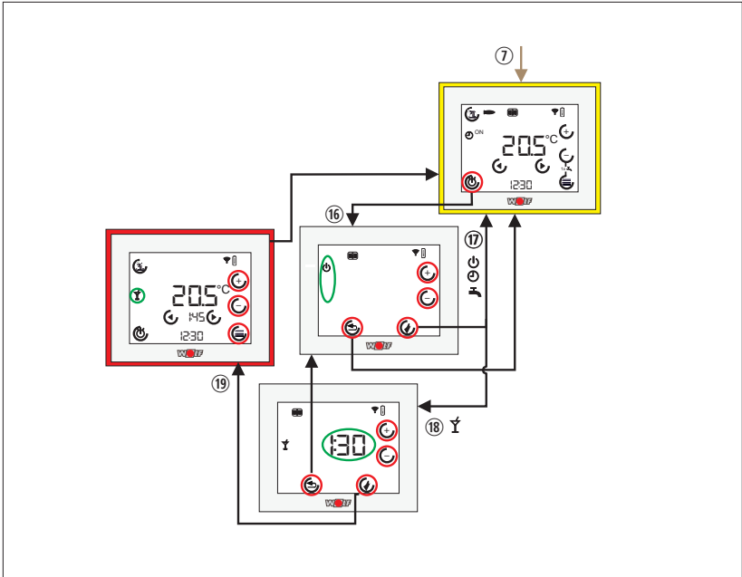
Рис. 10.10 Выбор программы
