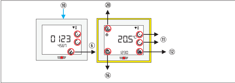
Рис. 10.3 Меню выбора
