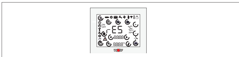
Рис. 6.1 Сброс
