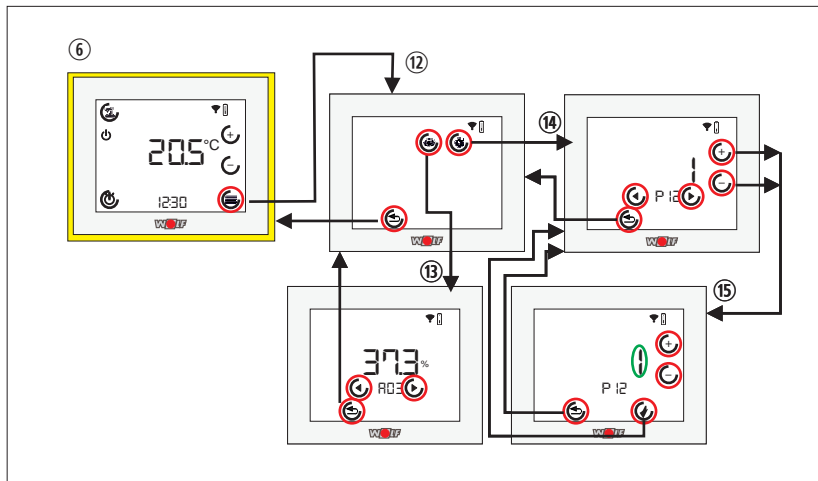
Рис. 10.5 Меню
